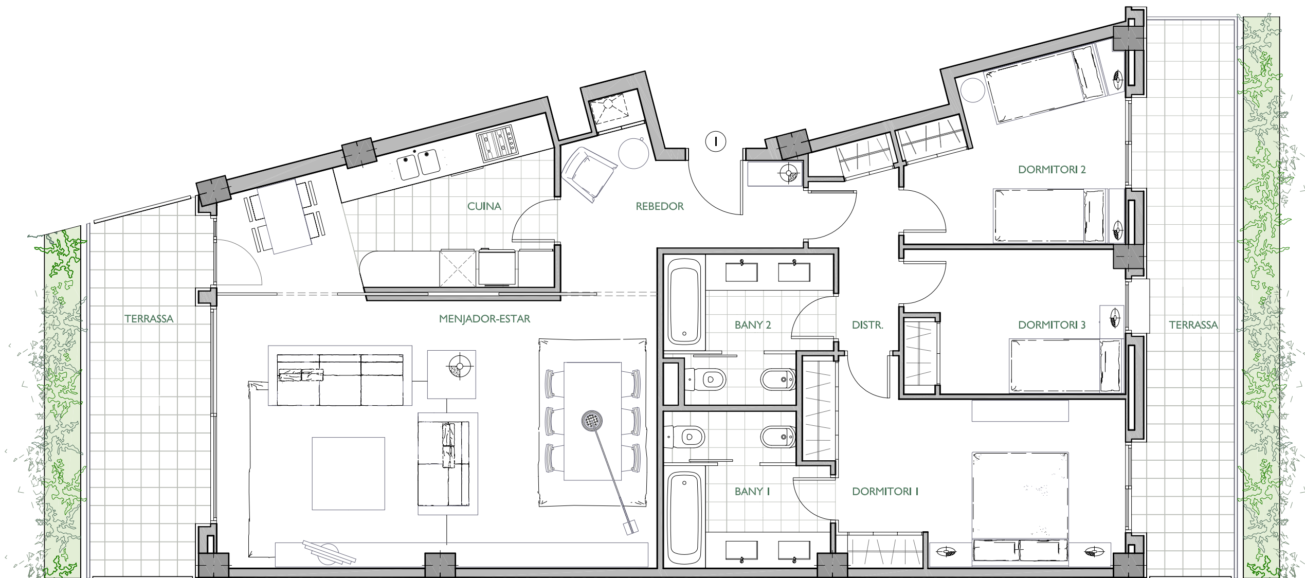
ESCALA B PLANTA PRIMERA - PORTA 1ª
