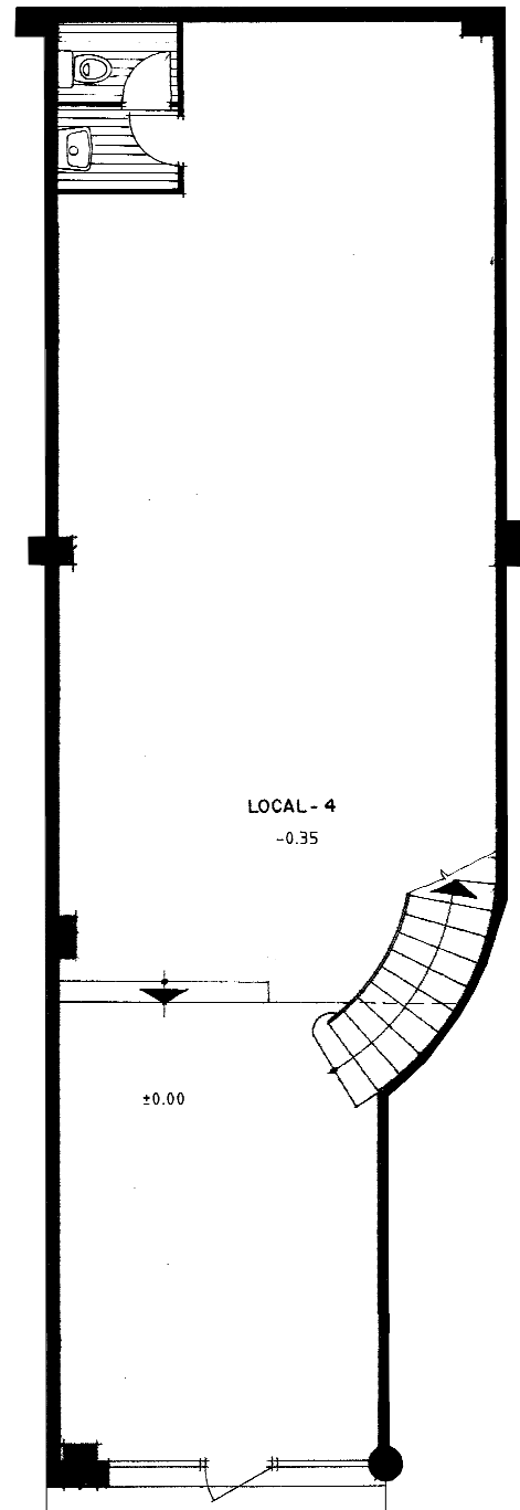
PLANTA BAIXA
