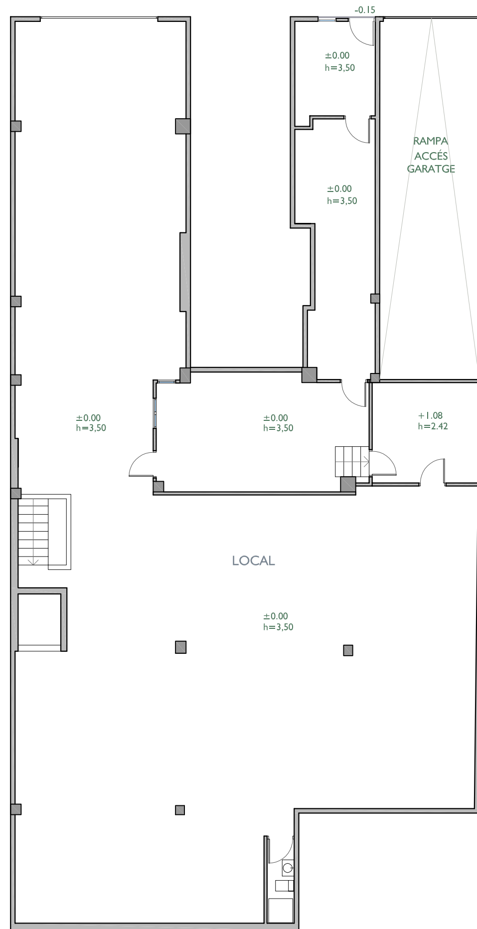
PLANTA BAIXA
