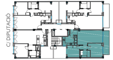
ESCALA I PLANTA QUARTA - PORTA 4ª
