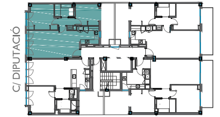
ESCALA I PLANTA CINQUENA - PORTA 2ª
