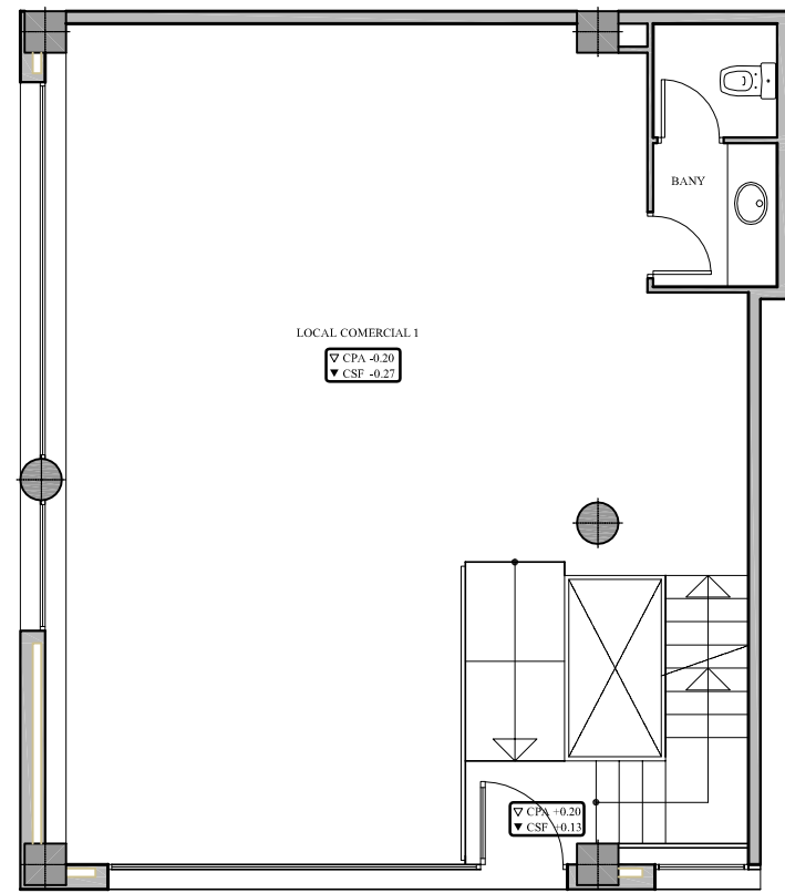
PLANTA BAIXA
