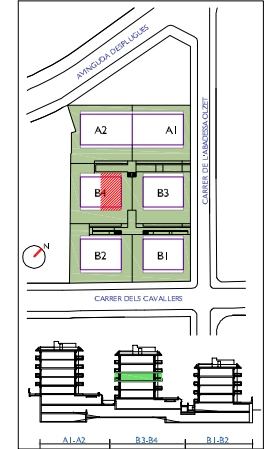
BLOC B4 PLANTA SEGONA - PORTA 2ª
