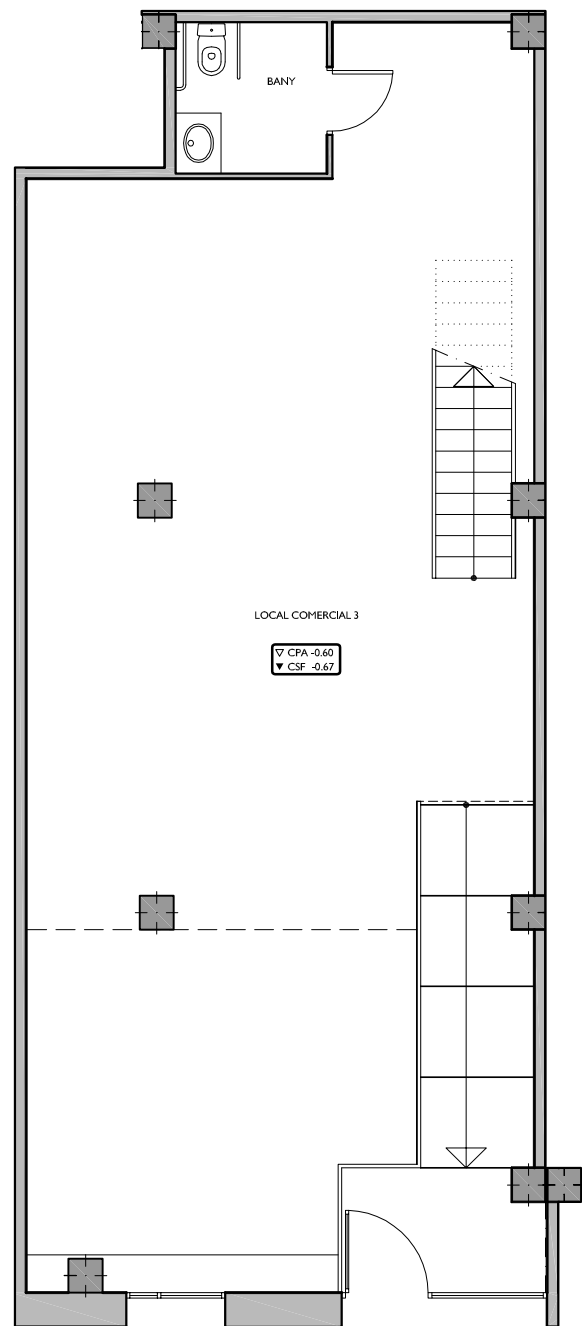
PLANTA BAIXA
