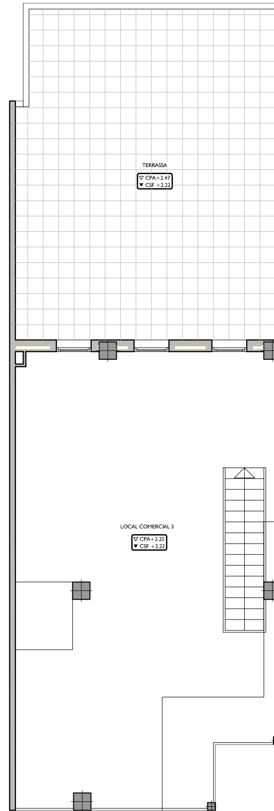
PLANTA ALTELL
