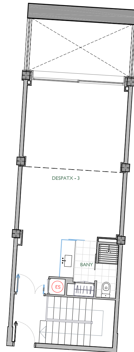
PLANTA BAIXA
