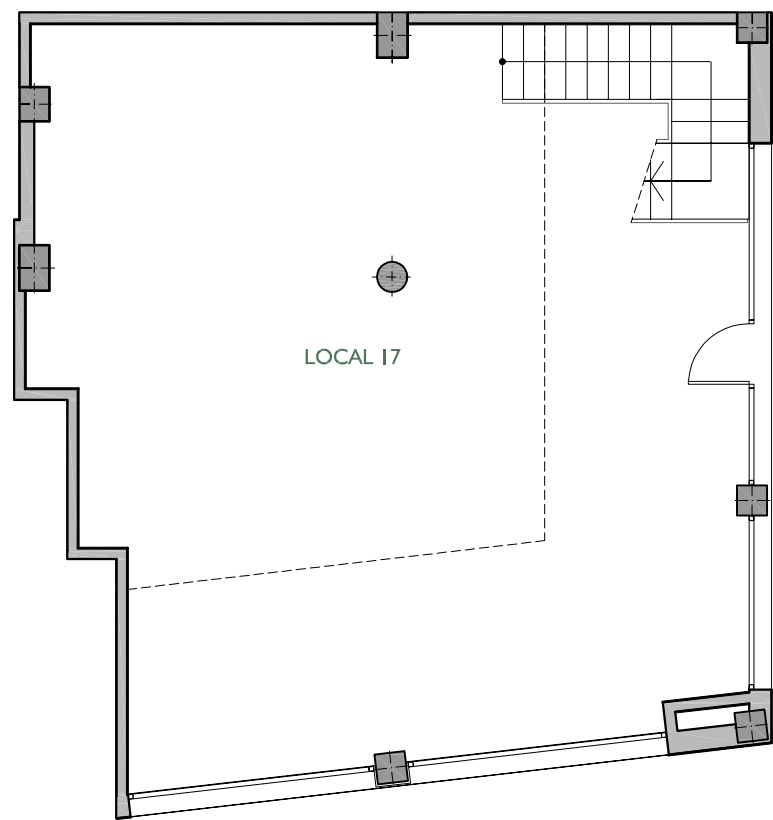
PLANTA BAIXA
