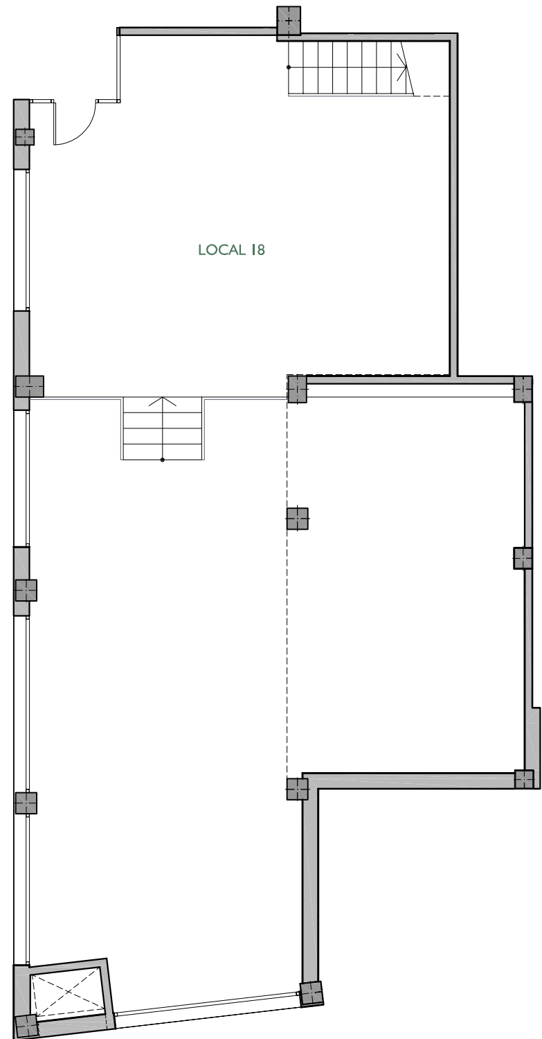
PLANTA BAIXA
