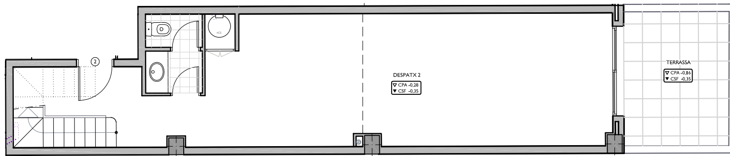
PLANTA BAIXA E:1/100
